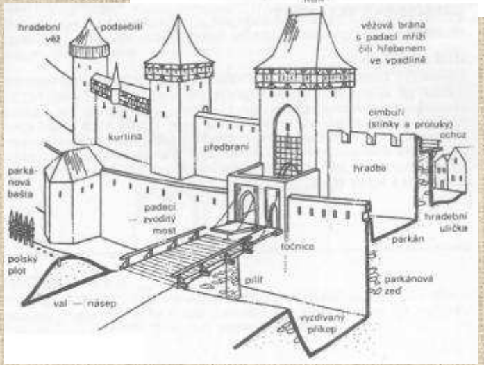
řez gotickým opevněním
