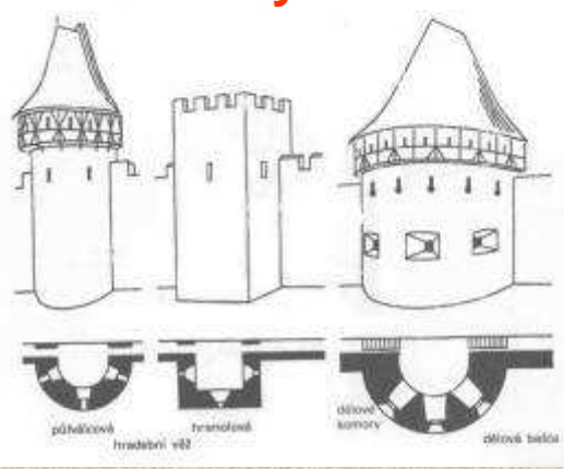
druhy bašt
