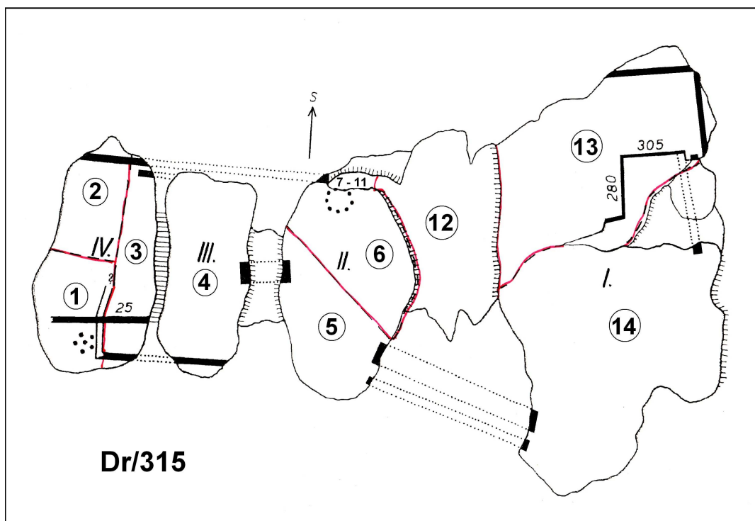
Obr. 27. Plán hradu Drábovna s vrcholně středověkými tesanými objekty (světnice, draže, ukotvení můstku). Pro potřeby projektu dokumentace skalních rytin byly vrcholové plošiny pracovně rozděleny na 14 poloh (desítky objektů souvisejících s turistickým ruchem). Skica bez měřítka. Podle J. Filipa 1947
