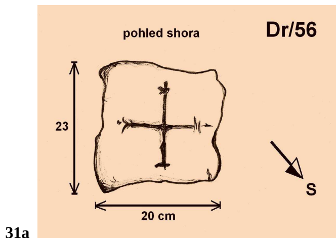
Obr. 31. Půdorysná skica historických hraničních kamenů v k. ú. Ondříkovice (Dr/56) a k. ú. Frýdštejn (Dr/262). Dokumentovali Z. Egertová, 2004 (31a) a Zdeněk Langr a Zbyšek Zdobinský, 2006 (31b)
